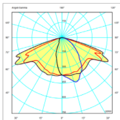
Diagramma polare esemplificativo. Distribuzione ottica stradale a richiesta.
