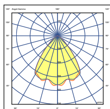
15LED 125W 700mA OTTICA 90°
