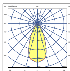
15LED 125W 700mA OTTICA 60°
